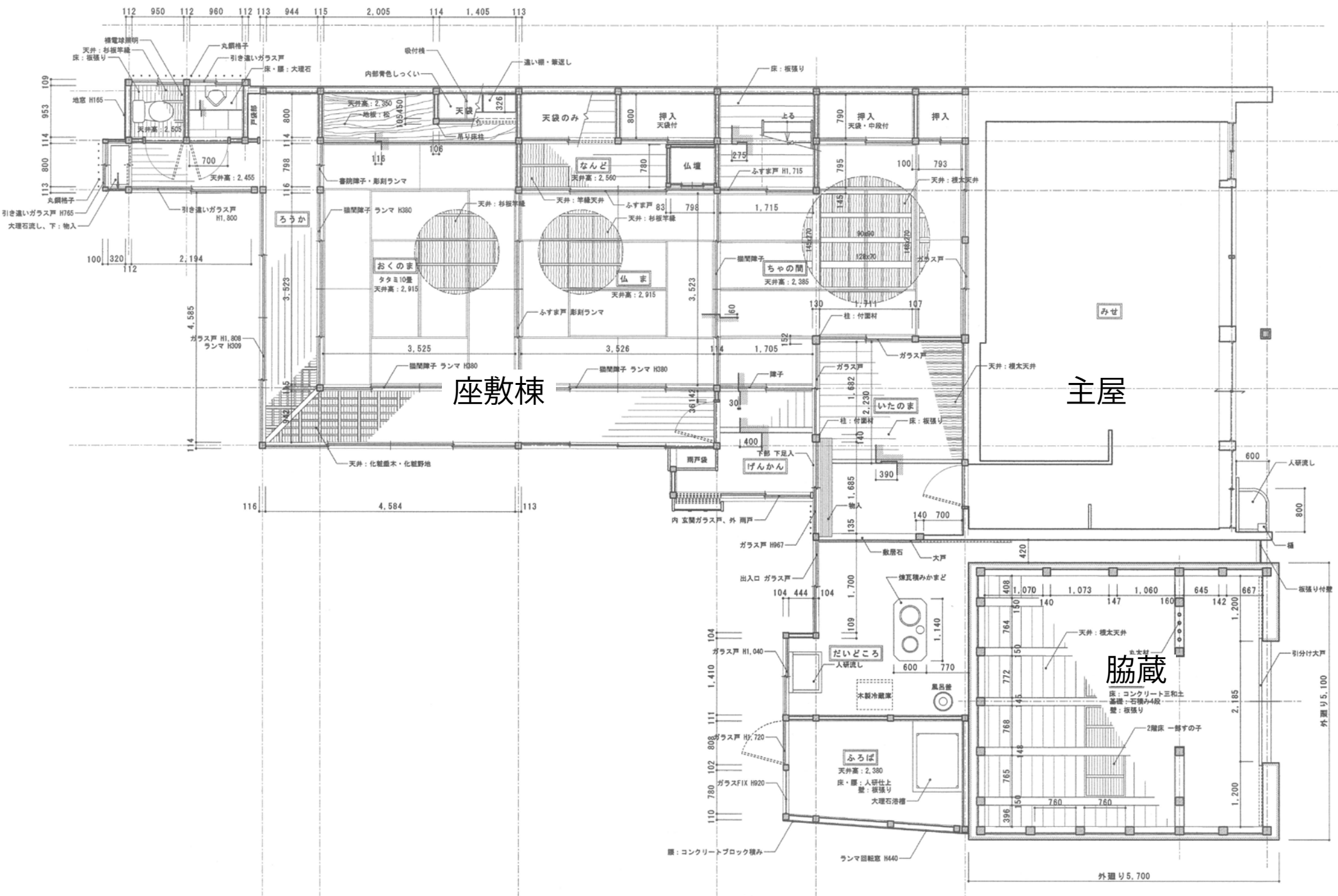
旧平井家住宅 1階平面図
