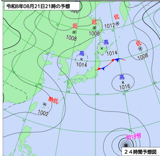
天気図予想 (21日21時)
