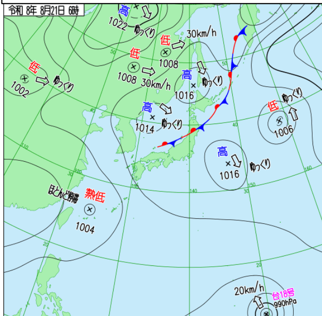
天気図実況 (21日06時)
