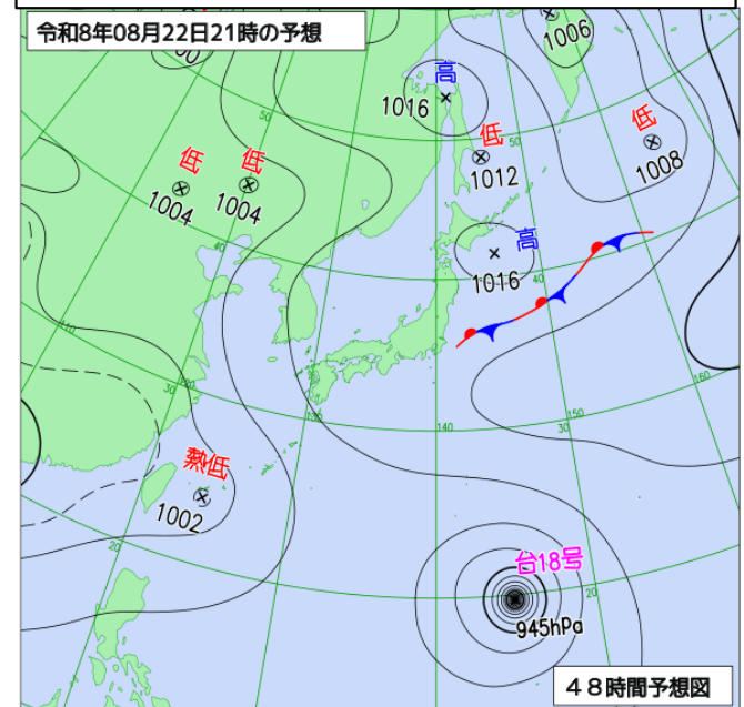
天気図予想 (22日21時)
