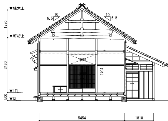
主屋見世現況梁間方向断面図 S=1/100
