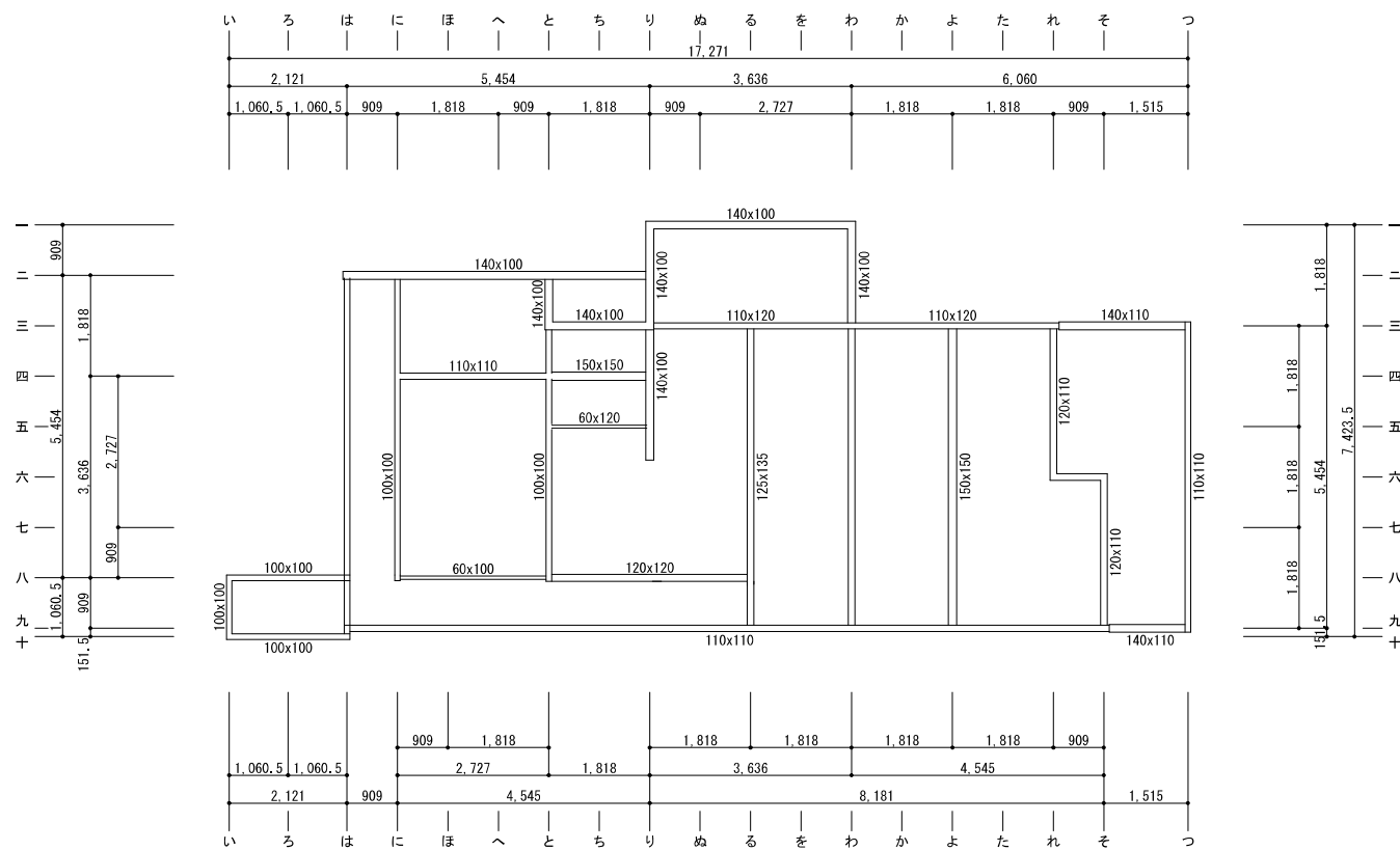
主屋現況床伏図 S=1/100
