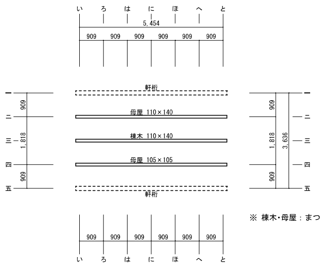
土蔵現況小屋伏図 S=1/100
