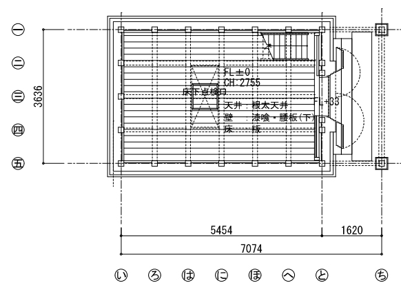
土蔵現況 1 階平面図 S=1/100
