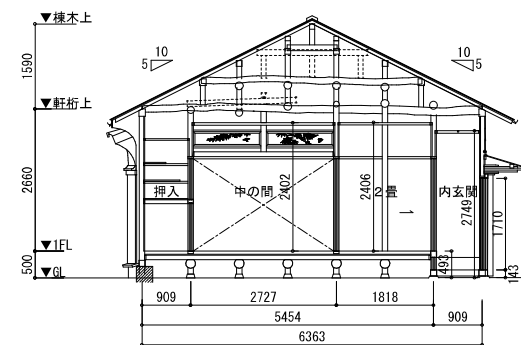
主屋中の間現況梁間方向断面図 S=1/100
