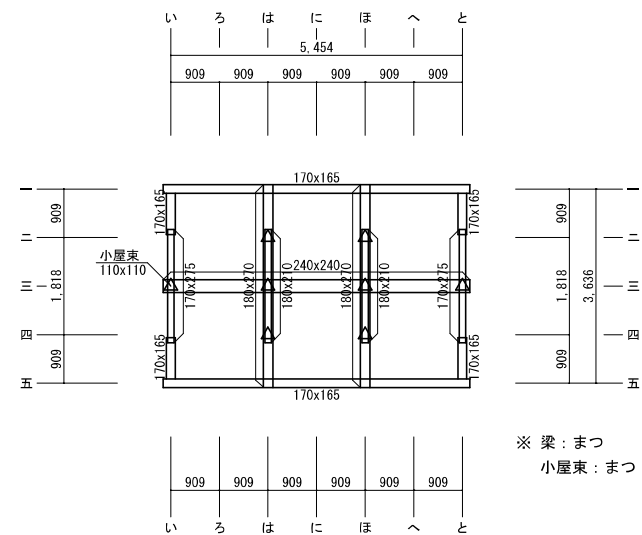
土蔵現況小屋梁伏図 S=1/100
