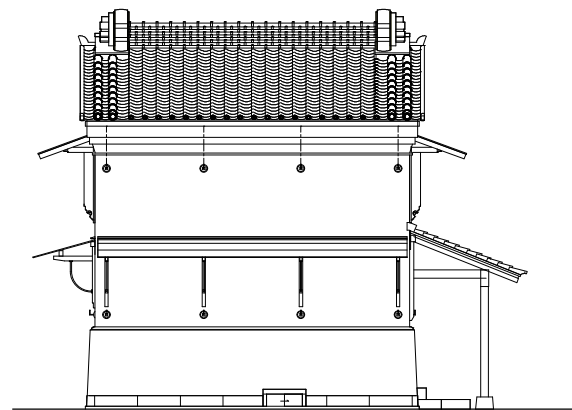
土蔵現況西面立面图 S=1/100
