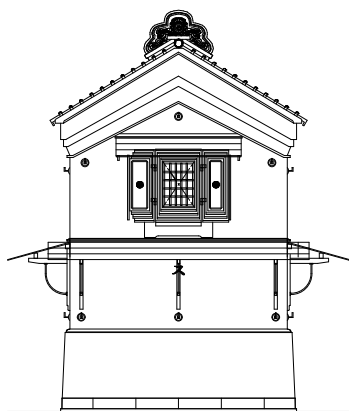
主屋現況北面立面图 S=1/100
