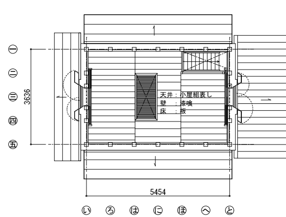
土蔵現況 2 階平面図 S=1/100
