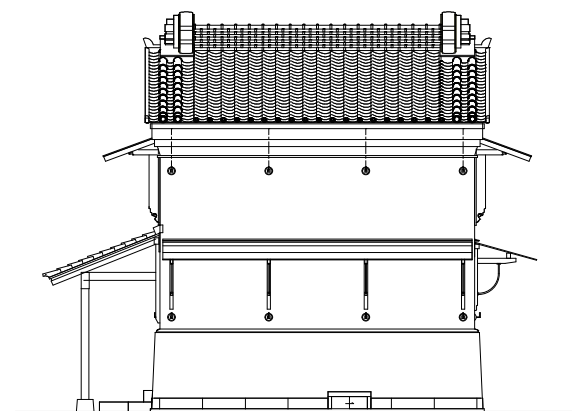
主屋現況東面立面图 S=1/100
