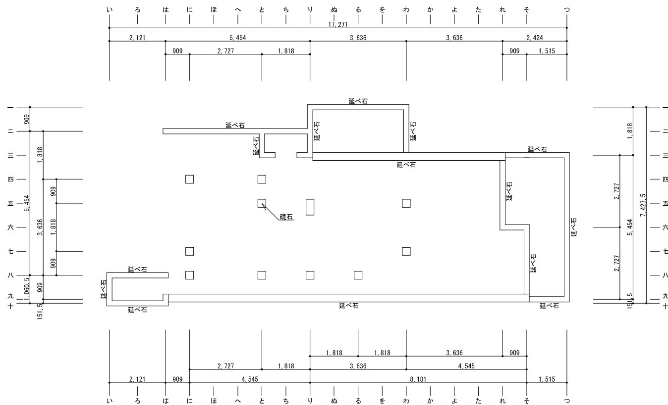
主屋現況基礎伏図 S=1/100
