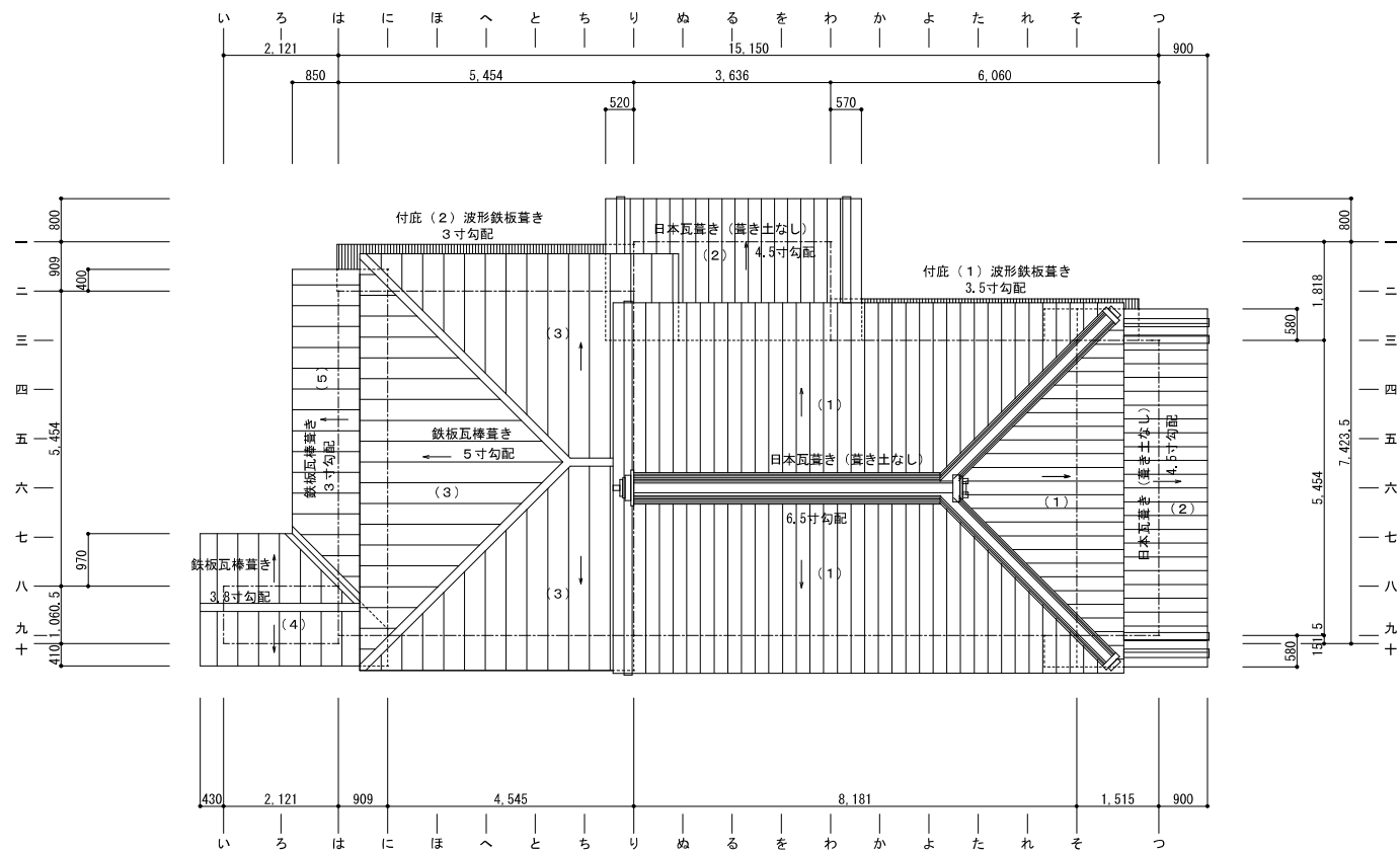
主屋現況屋根伏図 S=1/100
