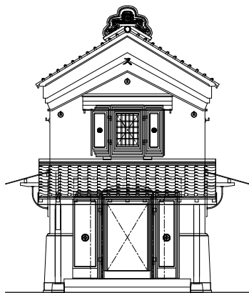
土蔵現況南面立面图 S=1/100
