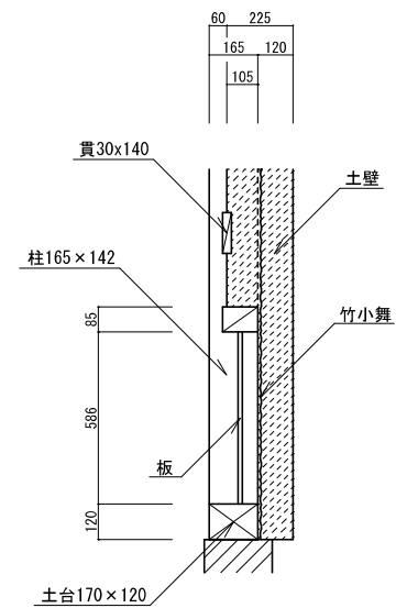
土蔵現況外壁断面詳細図 S=1/20
