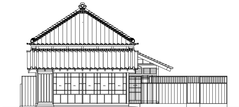
主屋現況南面立面図 S=1/100
