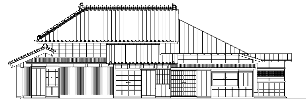
主屋現況東面立面図 S=1/100
