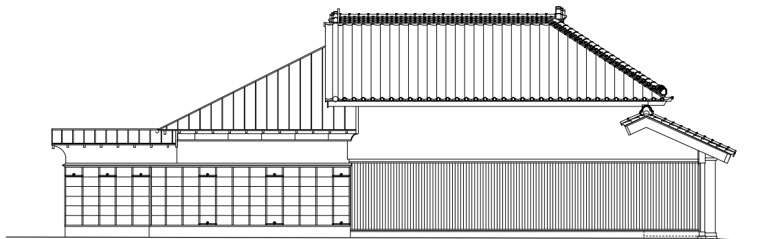
主屋現況西面立面図 S=1/100
