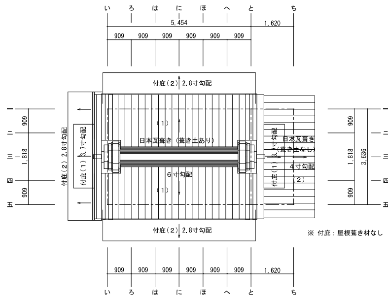
土蔵現況屋根伏図 S=1/100
