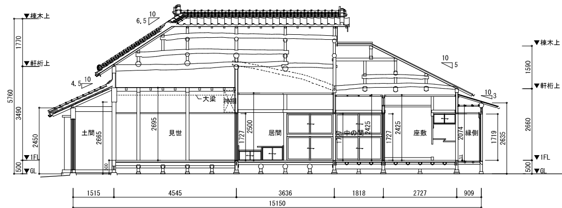
主屋現況桁行方向断面図 S=1/100
