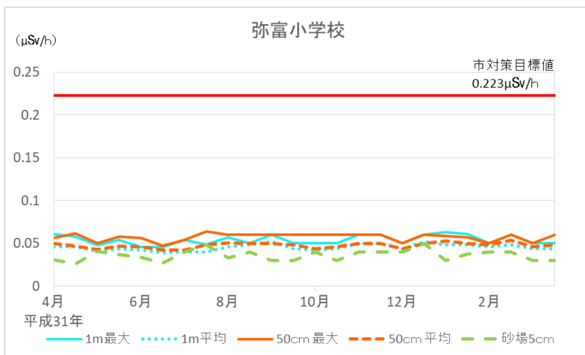
図 2-13-7 弥富小学校空間放射線量率の経月変化
