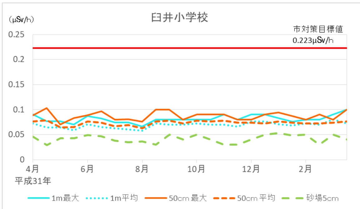
図 2-13-4 臼井小学校空間放射線量率の経月変化
