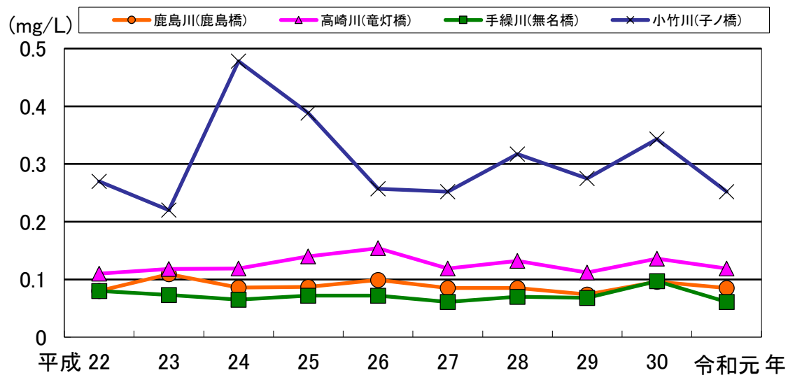
図 2-2-4 全リンの年平均値の経年変化
