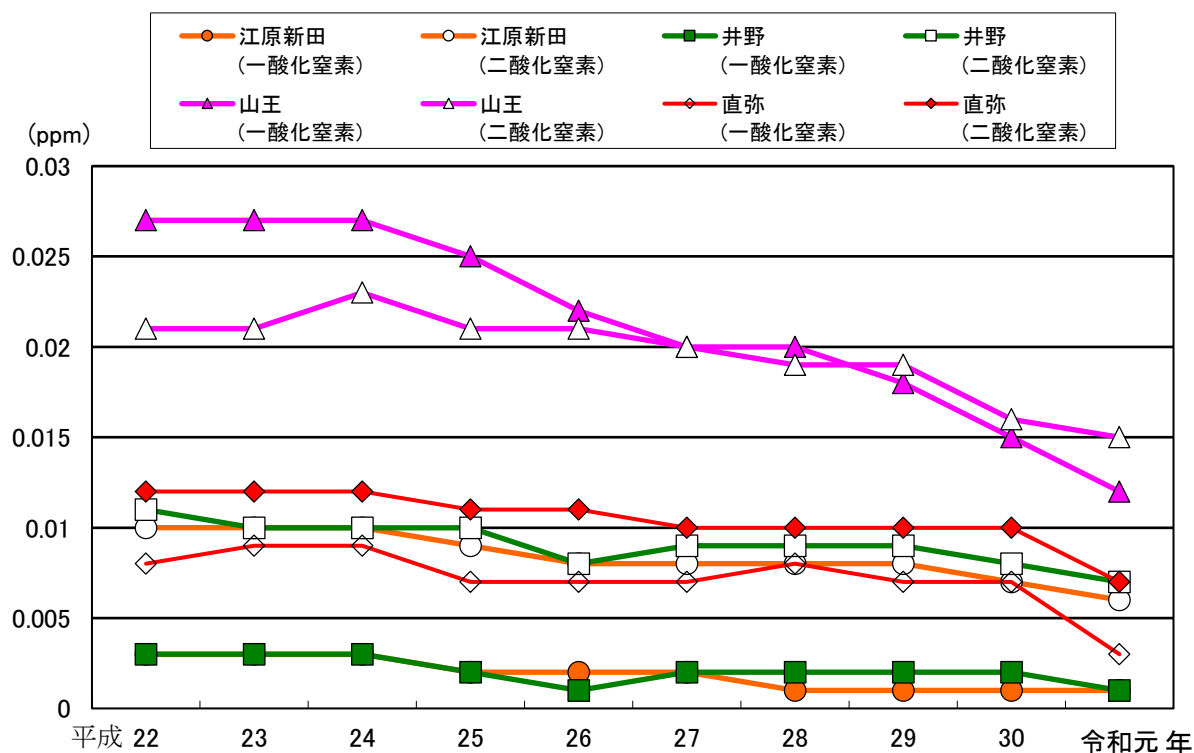
図 2-1-6 窒素酸化物濃度測定結果の年平均値の経年変化
