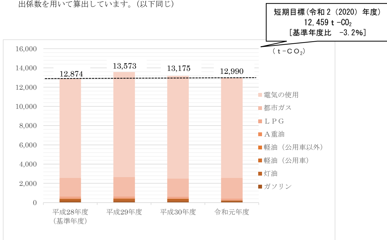
図2-12-3 全体の二酸化炭素排出量の推移
