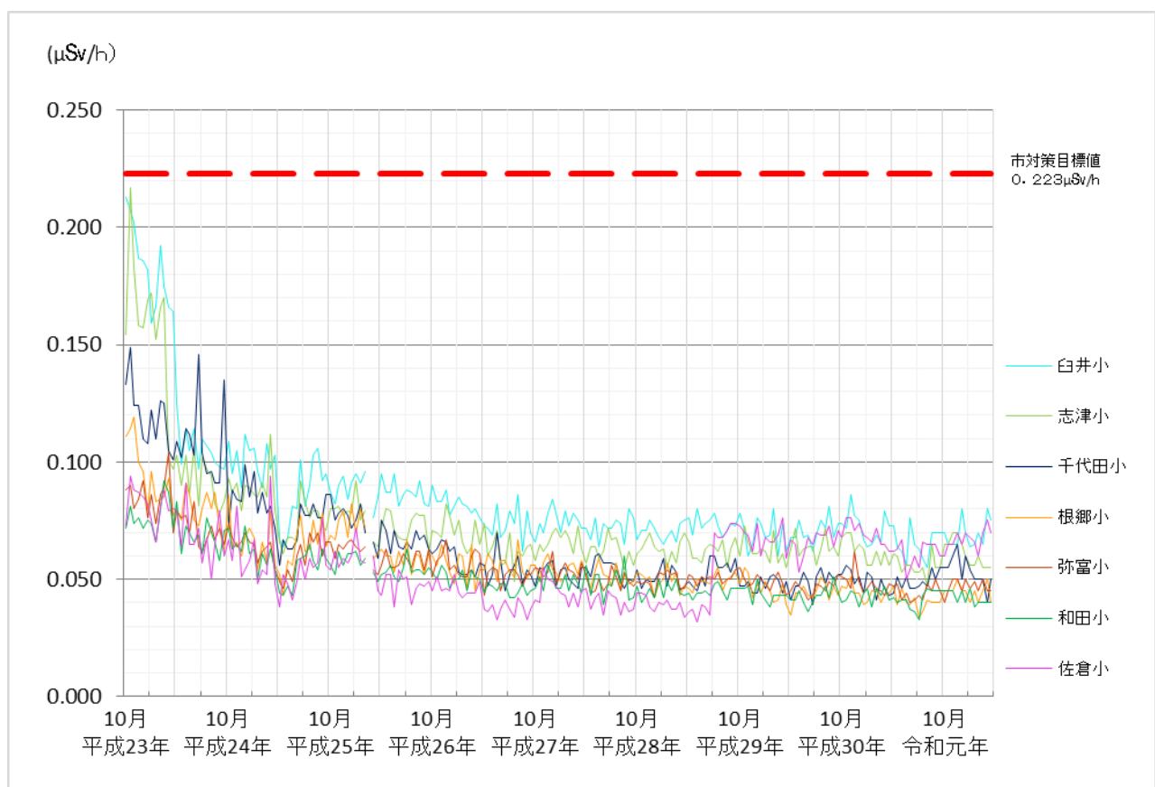
図 2-13-9 代表地点の空間放射線量率経年変化（中間値） ※月 2 回測定（平成 26 年 2 月のみ月 1 回測定）
