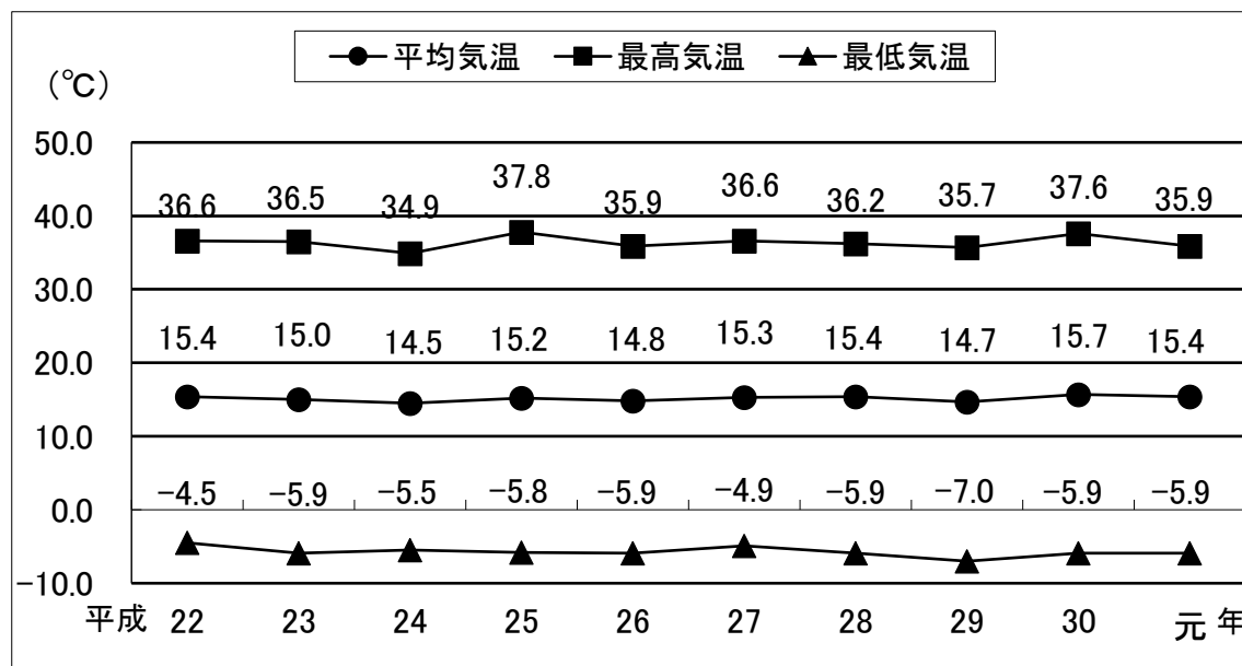
図 1-1-2 気温の経年変化 (出典) 令和 2 年版消防年報 佐倉市八街市酒々井町消防組合
