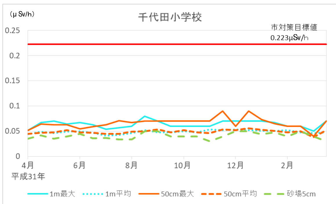
図 2-13-8 千代田小学校空間放射線量率の経月変化
