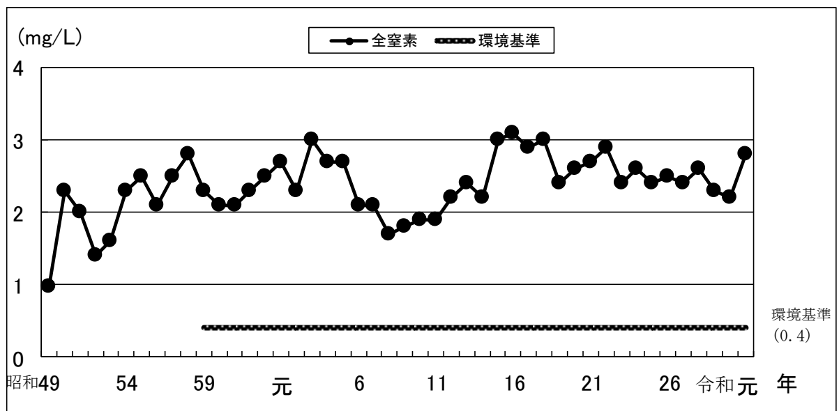
図 2-8-4 印旛沼の全窒素の年平均値
