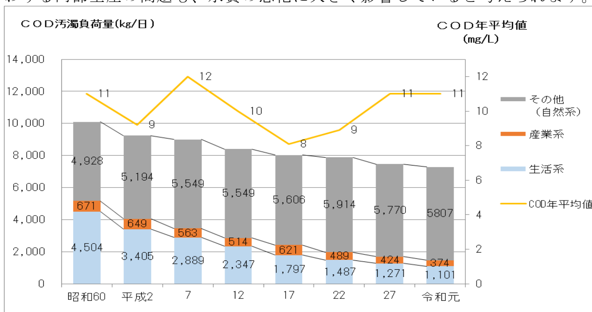
図 2-8-6 印旛沼のCOD発生源別汚濁負荷量・割合の変化
