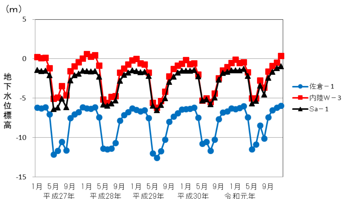
2-6-3 地下水位の経年変化
