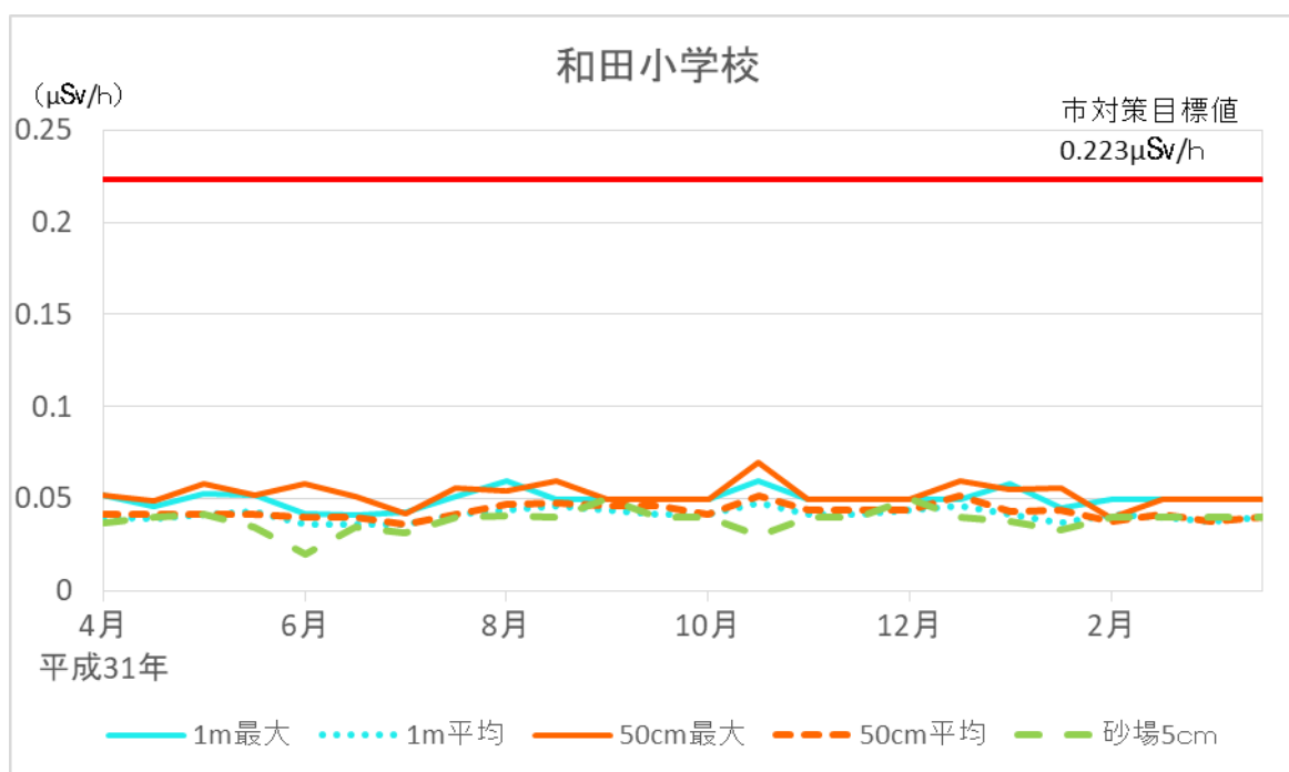
図 2-13-6 和田小学校空間放射線量率の経月変化
