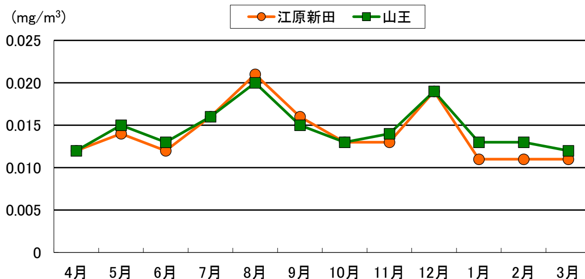
図2-1-10 令和元年度 浮遊粒子状物質濃度測定結果の月平均値の経月変化
