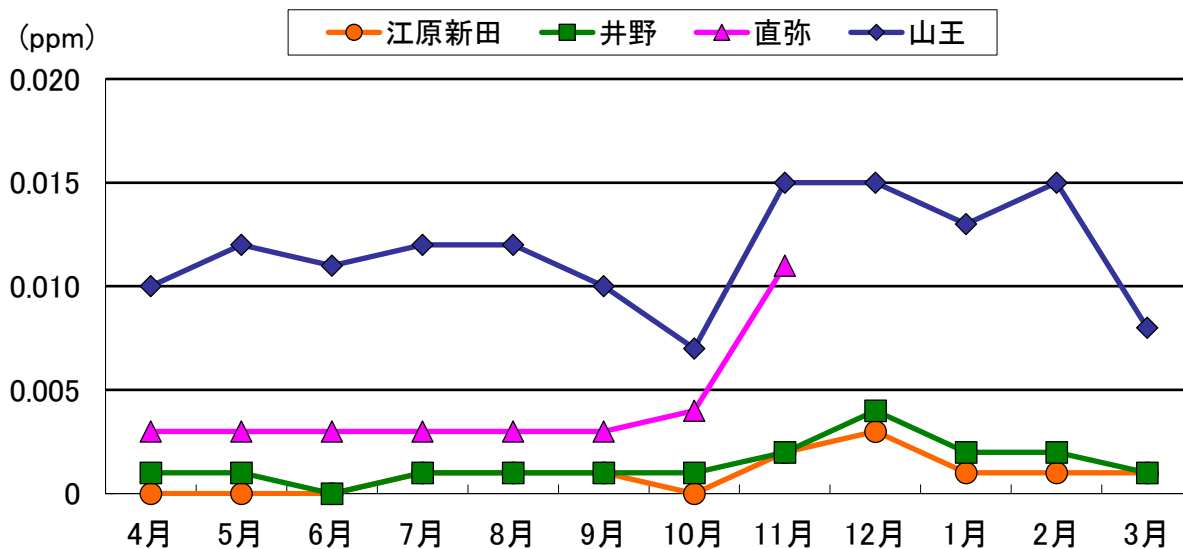
図2-1-4 令和元年度 一酸化窒素濃度測定結果の月平均値の経月変化
