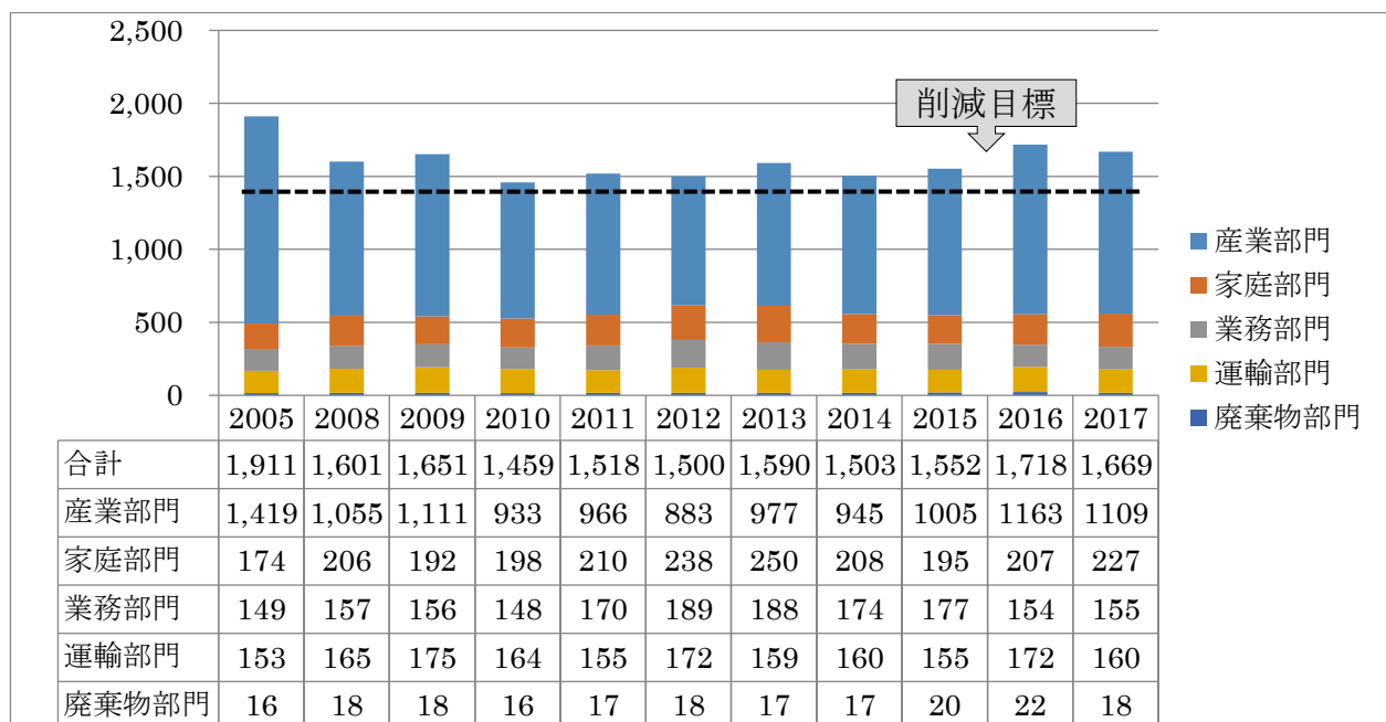
図 2-12-1 佐倉市から排出される二酸化炭素量推移 排出量 (千 t-CO2)
