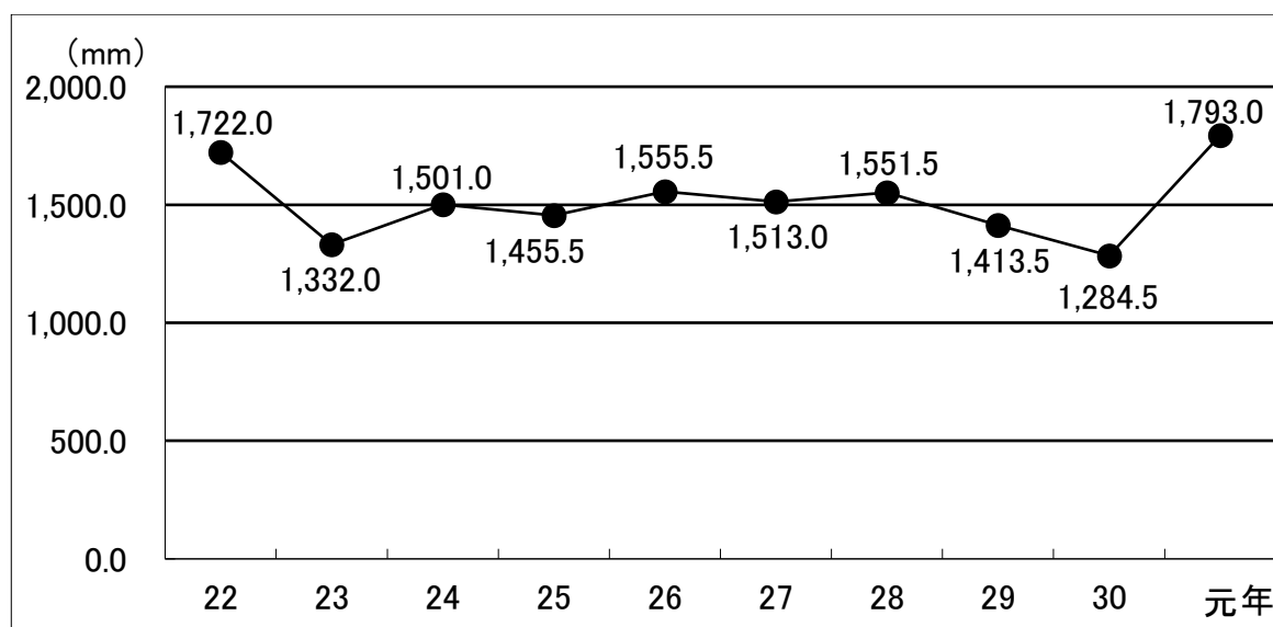
図 1-1-3 年間降水量の経年変化 (出典) 令和 2 年版消防年報 佐倉市八街市酒々井町消防組合
