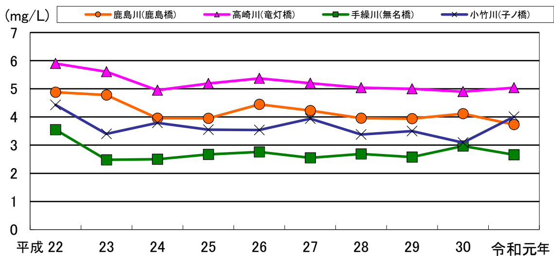
図 2-2-3 全窒素の年平均値の経年変化
