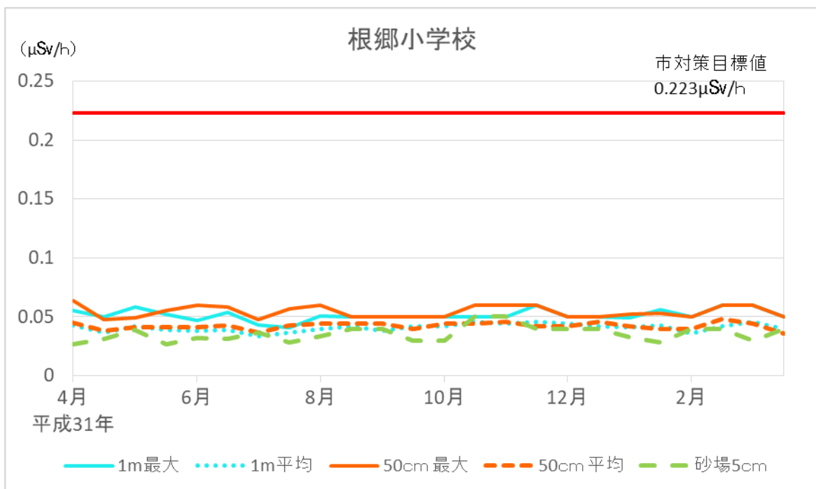
図 2-13-5 根郷小学校空間放射線量率の経月変化
