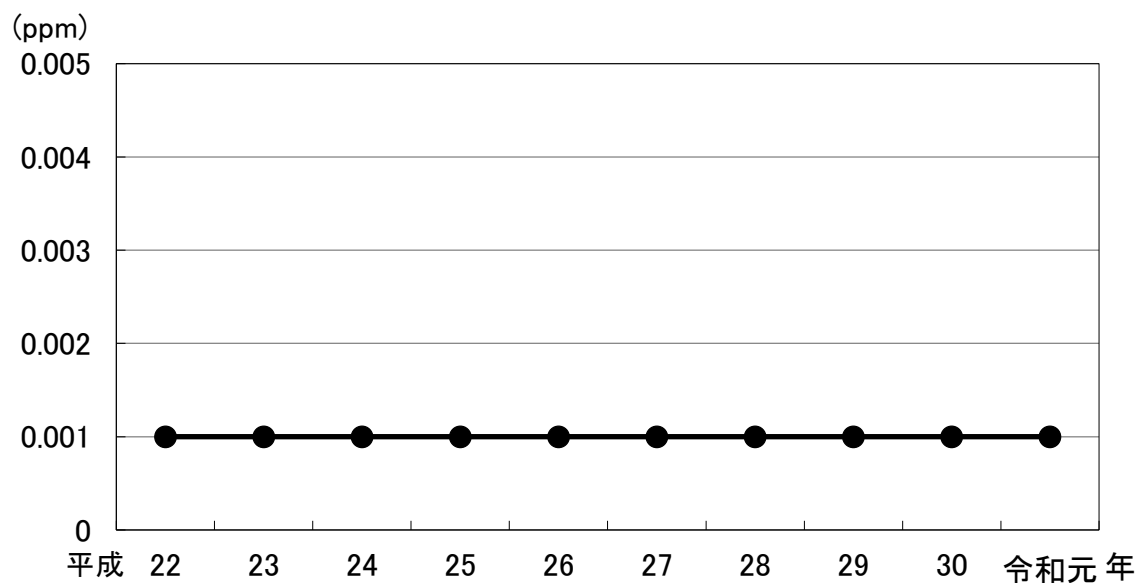
図 2-1-3 二酸化硫黄濃度測定結果の年平均値の経年変化
