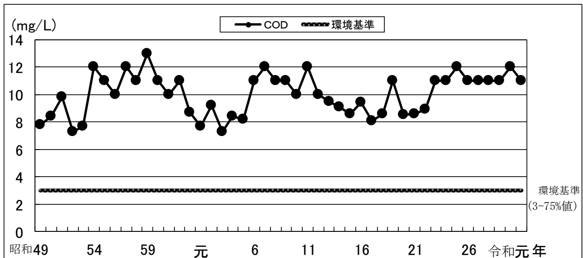
図 2-8-3 印旛沼 C O D の年平均値
