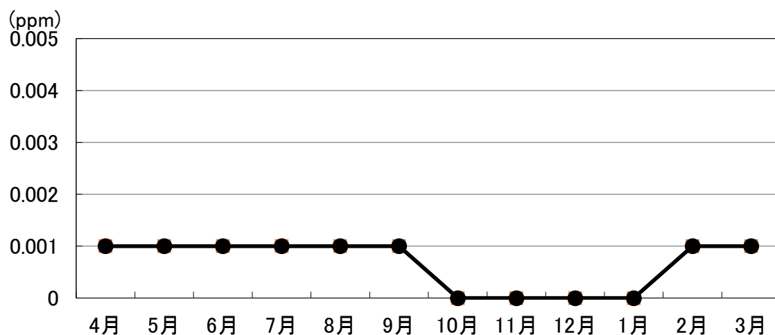
図 2-1-2 令和元年度 二酸化硫黄濃度測定結果の月平均値の経月変化
