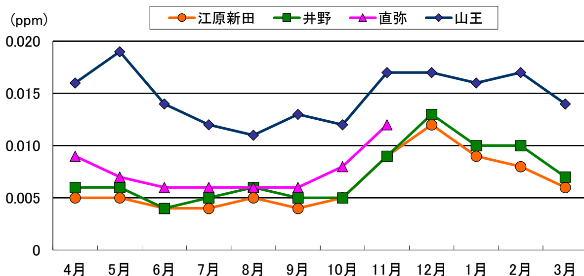
図 2-1-5 令和元年度 二酸化窒素濃度測定結果の月平均値の経月変化
