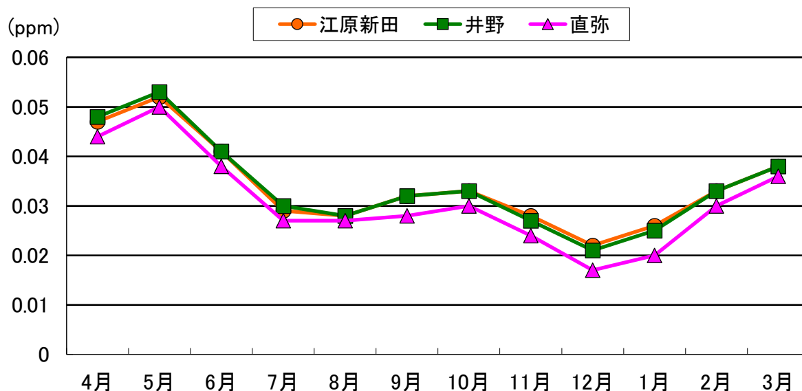
図2-1-7 令和元年度 光化学オキシダント濃度測定結果の月平均値の経月変化
