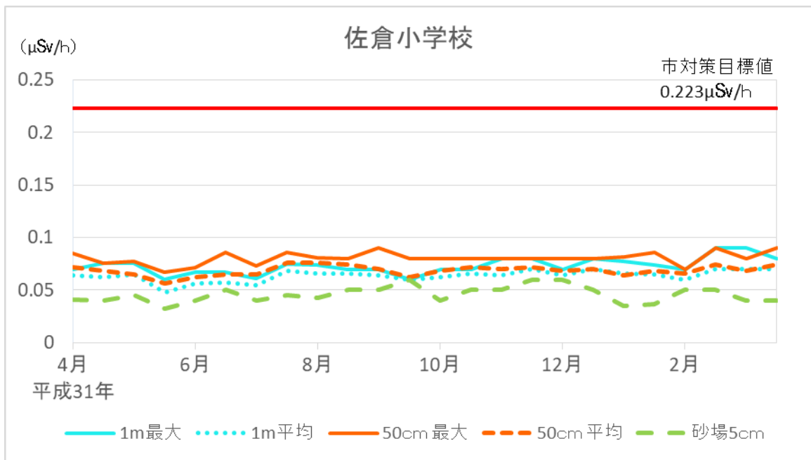
図 2-13-2 佐倉小学校空間放射線量率の経月変化
