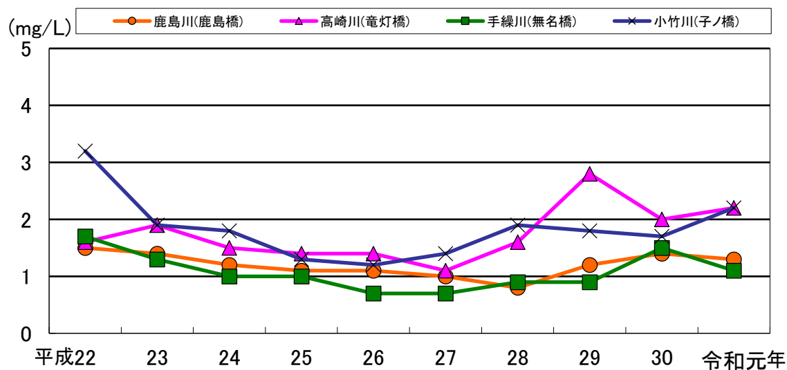
図 2-2-2 BODの年平均値の経年変化
