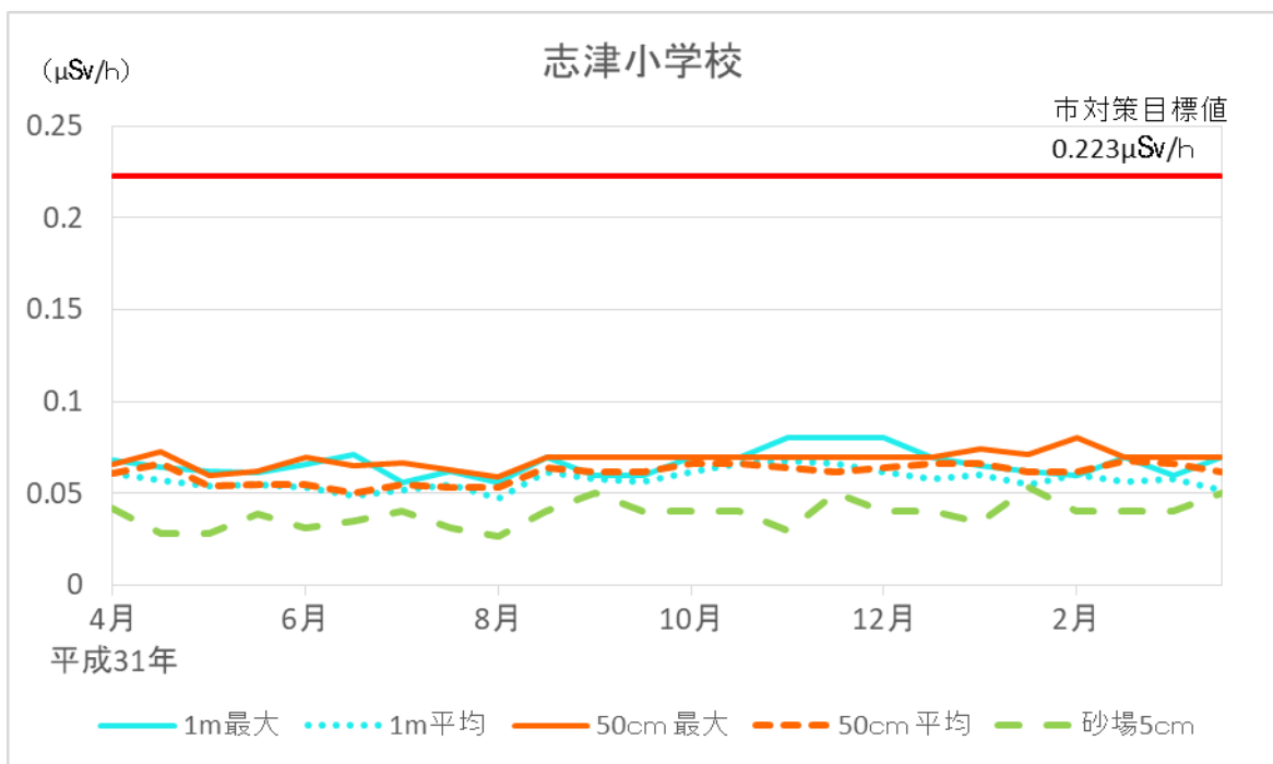
図 2-13-3 志津小学校空間放射線量率の経月変化
