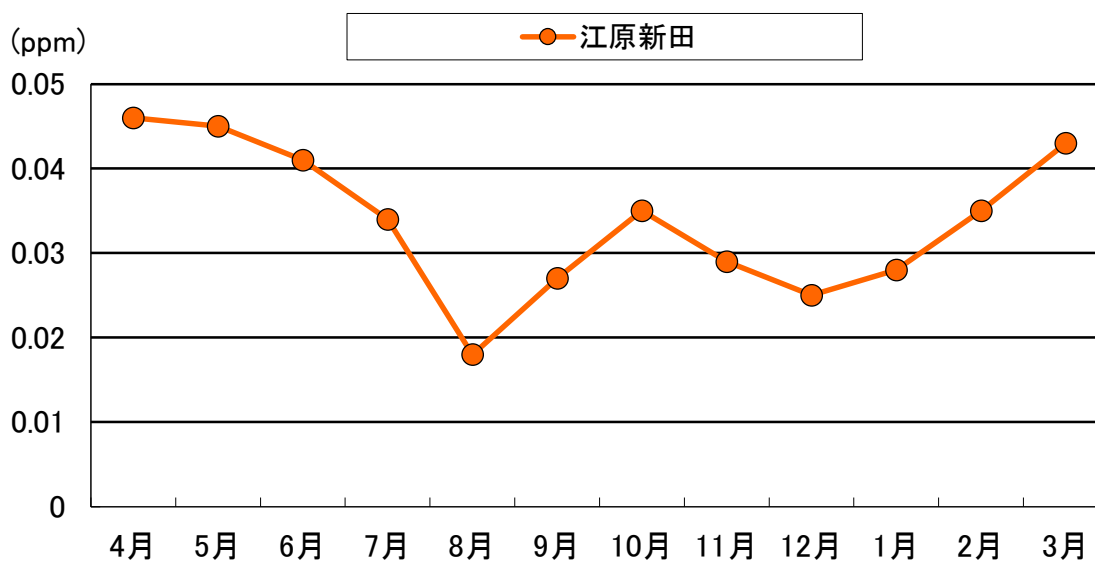
図 2-1-7 令和 5 年度 光化学オキシダント濃度測定結果の月平均値の経月変化
