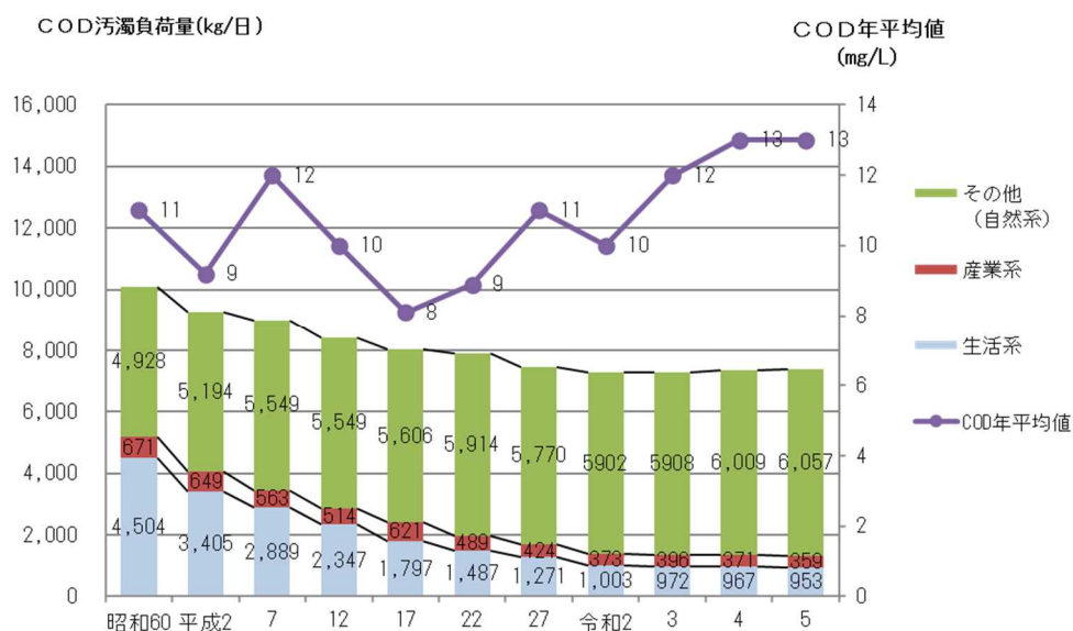
図 2-8-6 印旛沼の COD 発生源別汚濁負荷量・割合の変化
