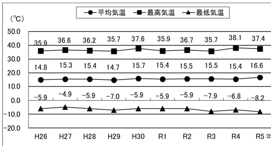
図 1－1－2 気温の経年変化
