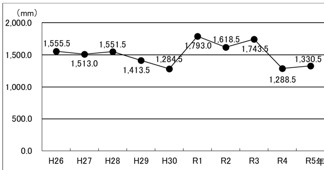
図 1-1-3 年間降水量の経年変化 (出典) 気象庁
