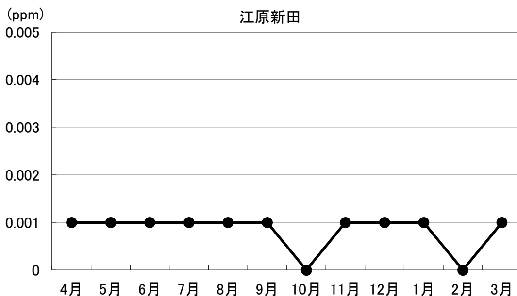
図 2-1-2 令和 5 年度 二酸化硫黄濃度測定結果の月平均値の経月変化
