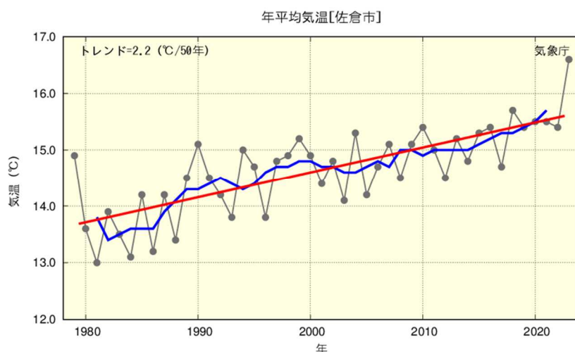
図 2-12-4 佐倉市の年平均気温の経年変化（銚子地方気象台提供）
