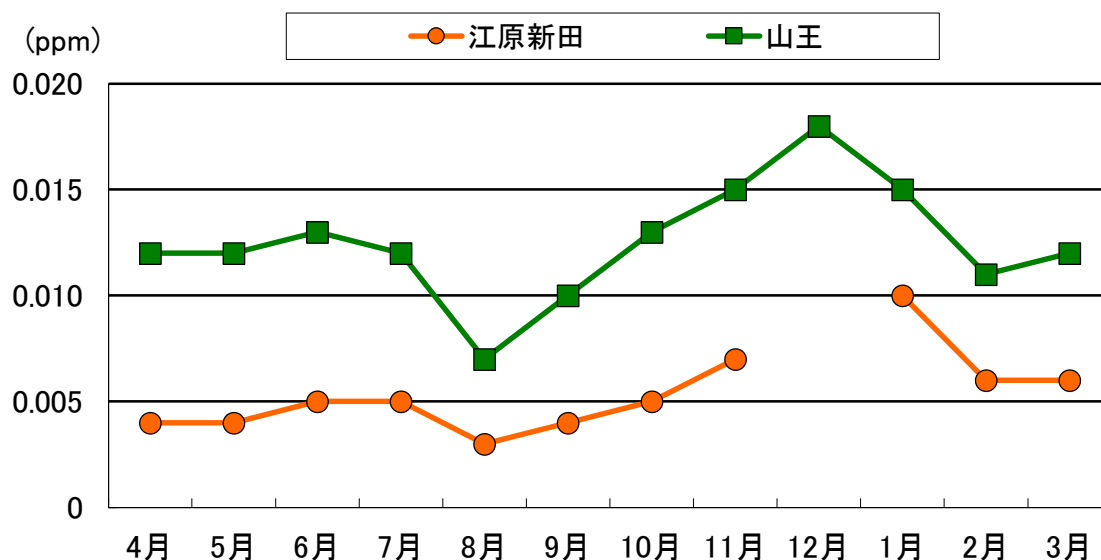
図 2-1-5 令和 5 年度 二酸化窒素濃度測定結果の月平均値の経月変化
