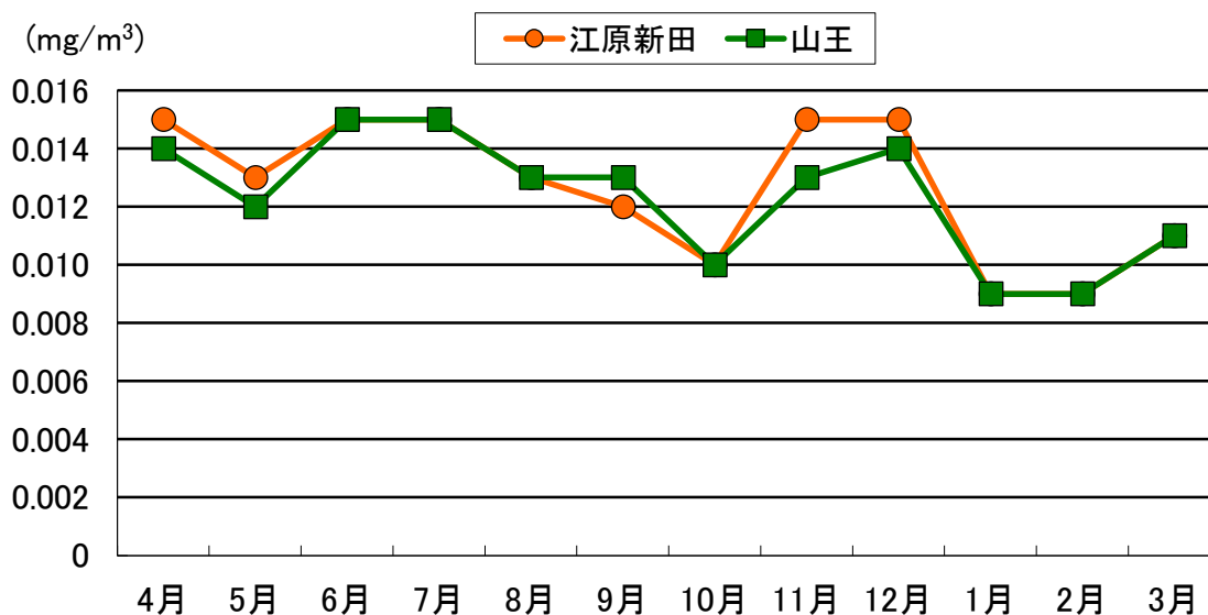
図2-1-10 令和5年度 浮遊粒子状物質濃度測定結果の月平均値の経月変化
