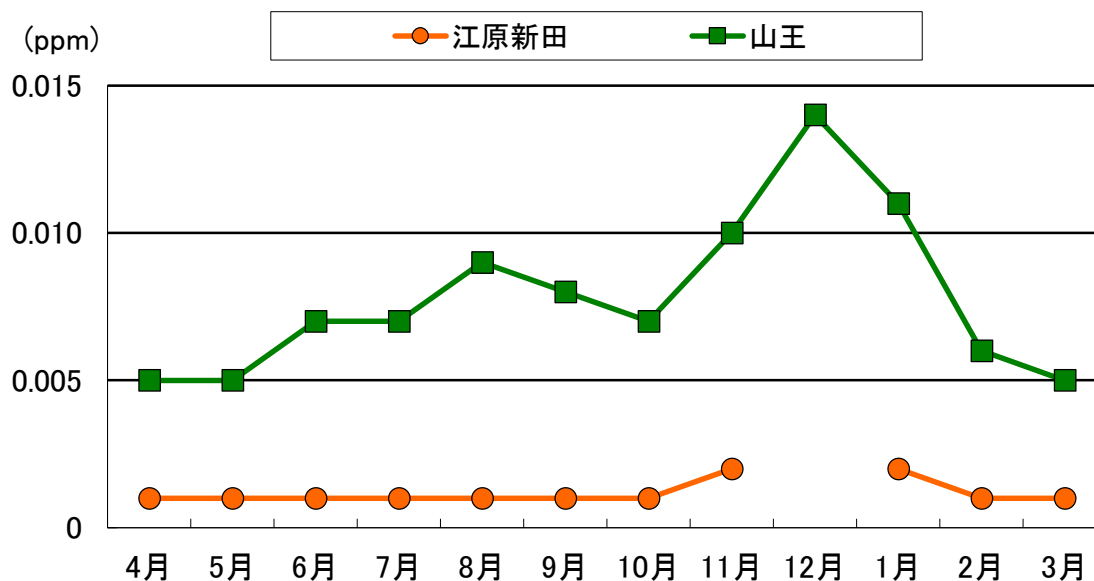
図2-1-4 令和5年度 一酸化窒素濃度測定結果の月平均値の経月変化
