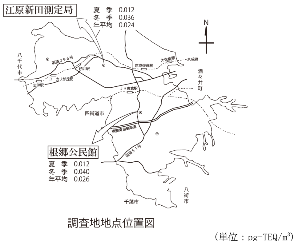
図2-10-1 大気環境中のダイオキシン類調査位置及び結果図
