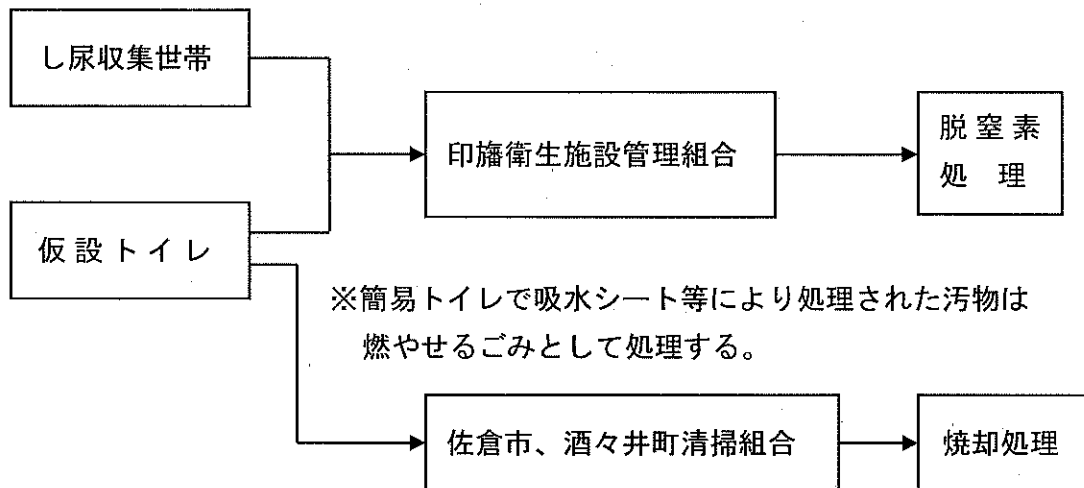
図4 処理フロー
