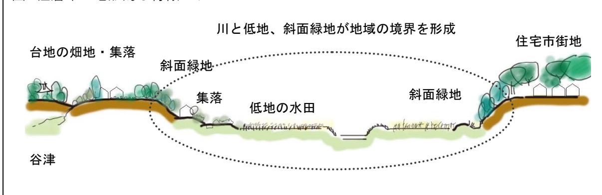
図 佐倉市の地形的な特徴のイメージ
