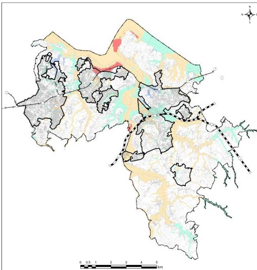
図 液状化想定（東京湾北部地震）
