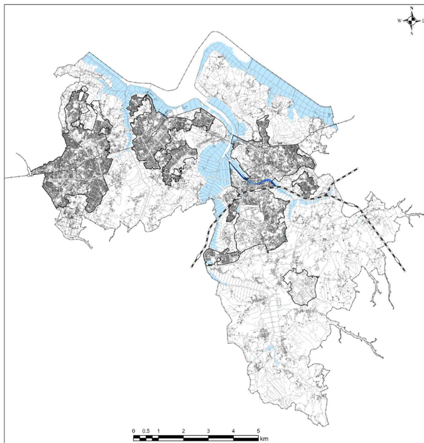
図 長期浸水（3日以上）区域、家屋倒壊等氾濫想定区域
