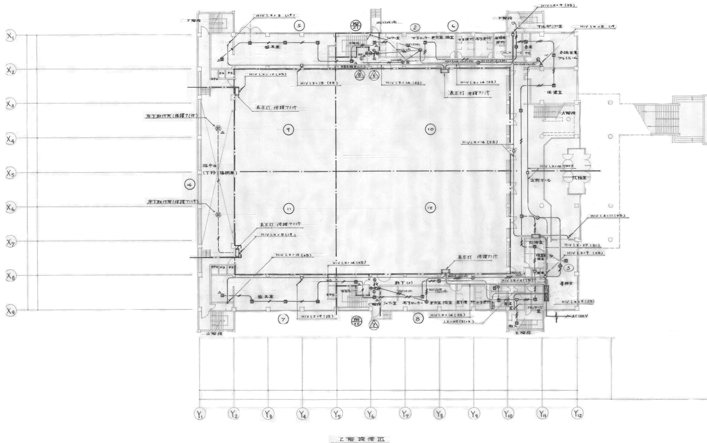
2階設備図
