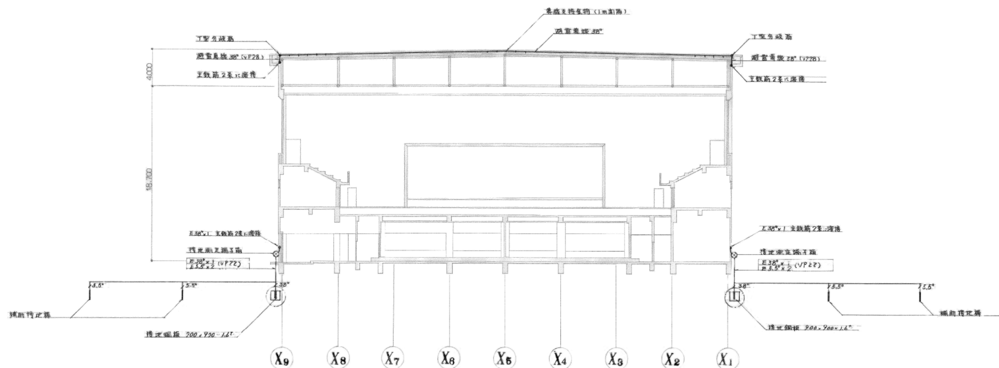
西側立面図
