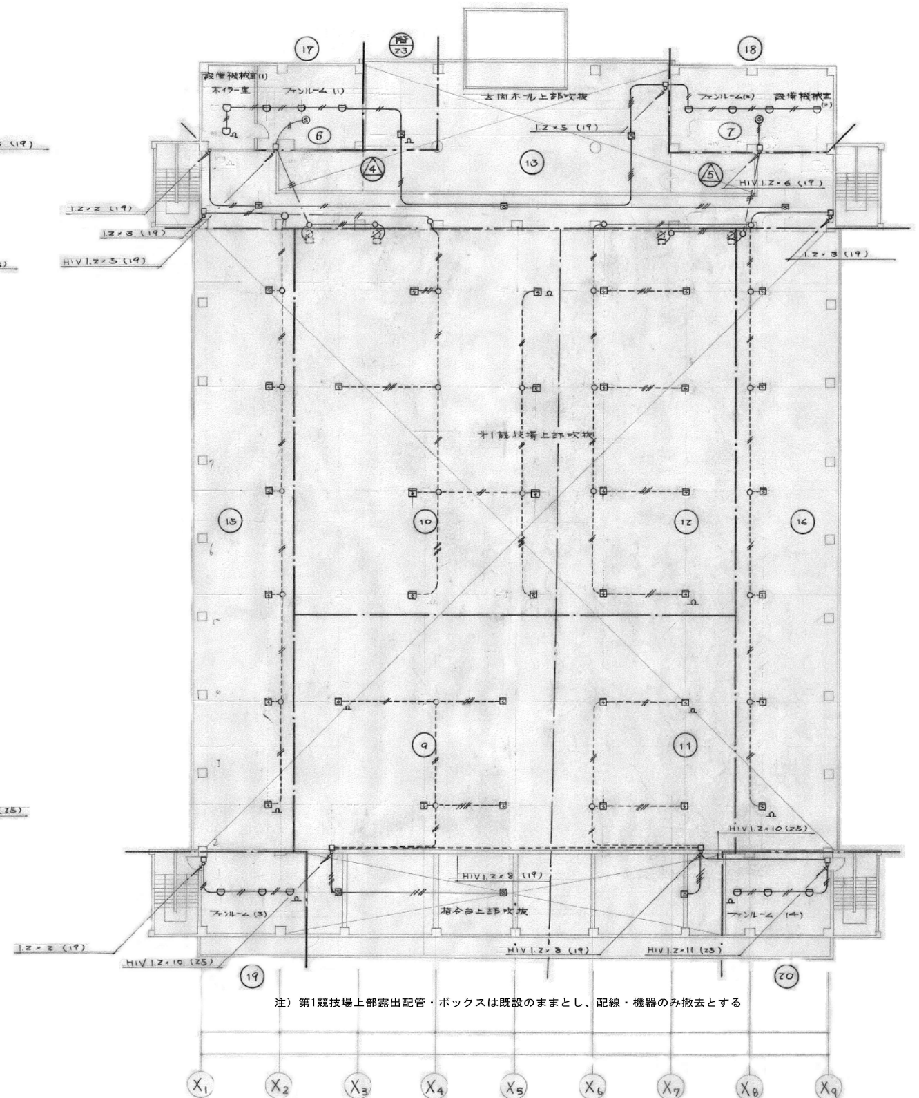
4階設備図
