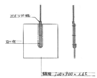
接地銅板
