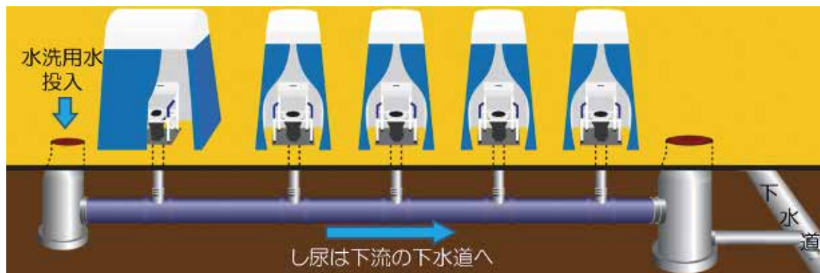
▲マンホールトイレの仕組み
