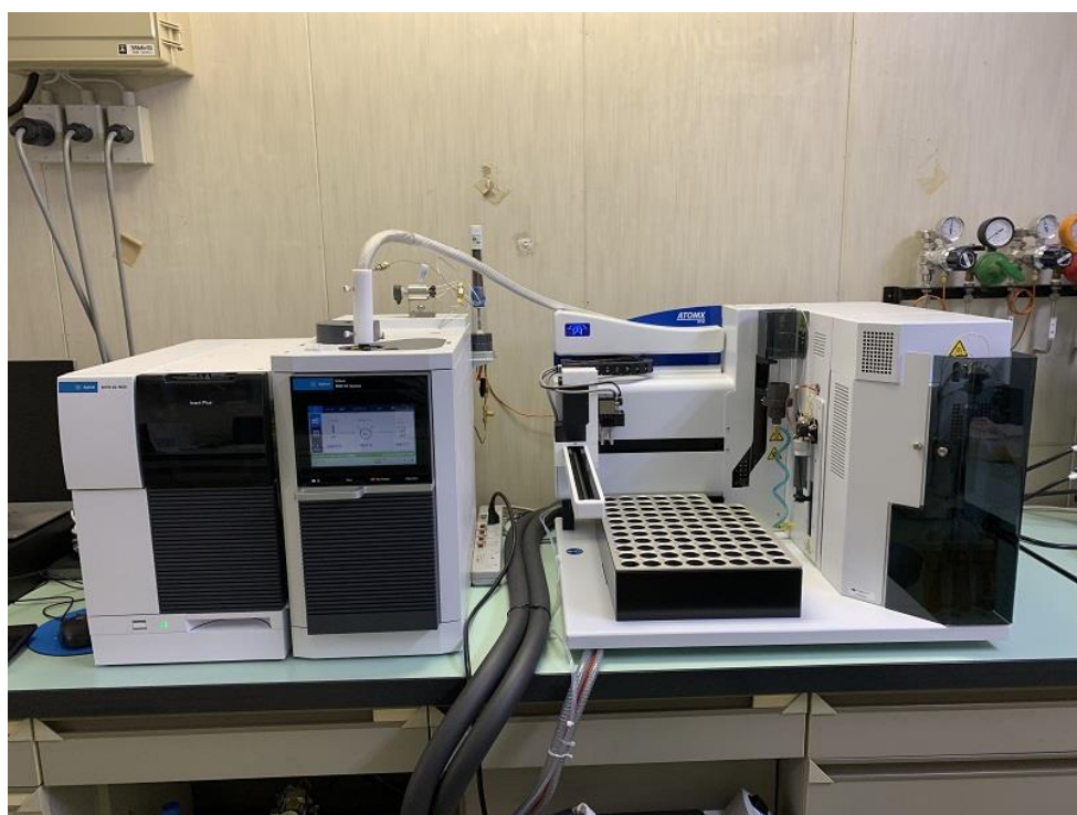
ガスクロマトグラフ質量分析装置
