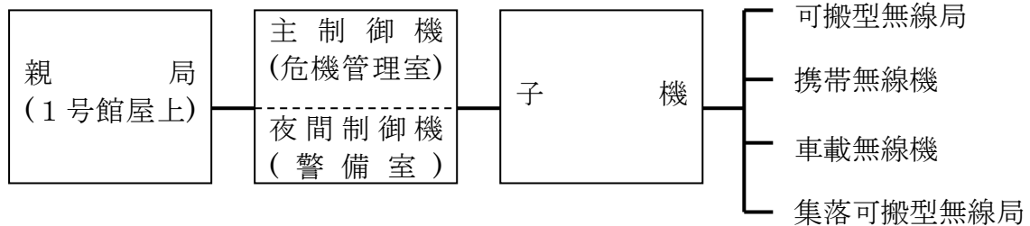
【防災行政無線（移動系）系統図】
